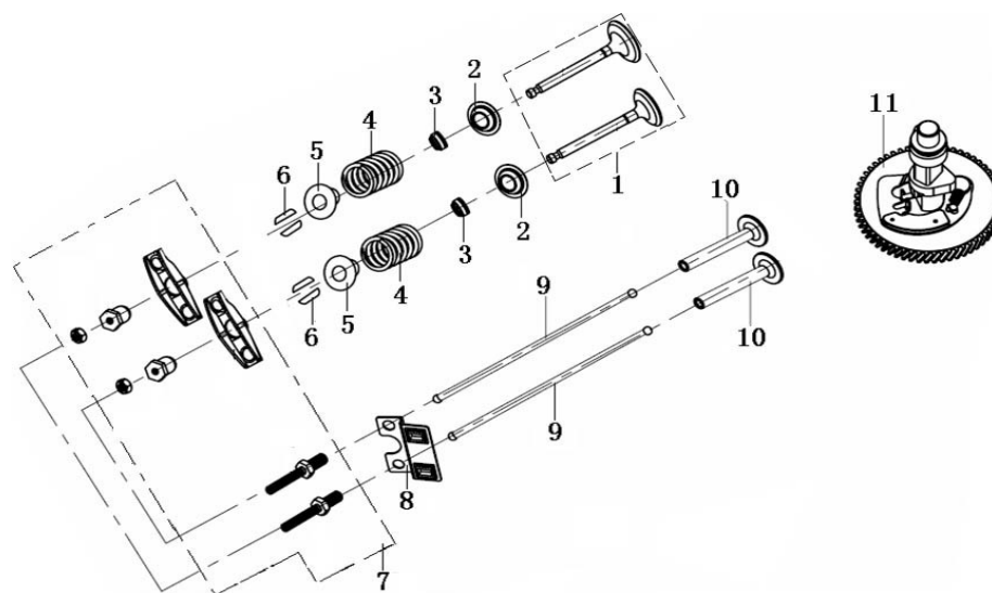
配气机构 (Valve)
